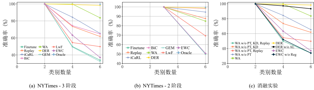
图9 不同类别增量学习算法在新闻分类数据集 NYTimes 上的实验分析
