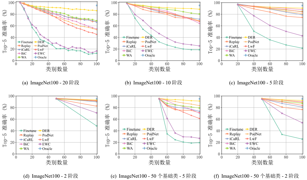
图6 增量学习算法在 ImageNet100 数据集上的 Top-5 准确率
