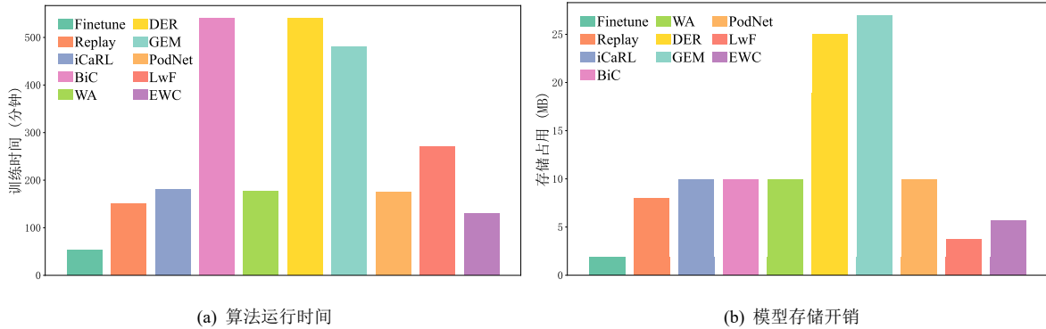
图7 运行时间和模型存储开销对比
