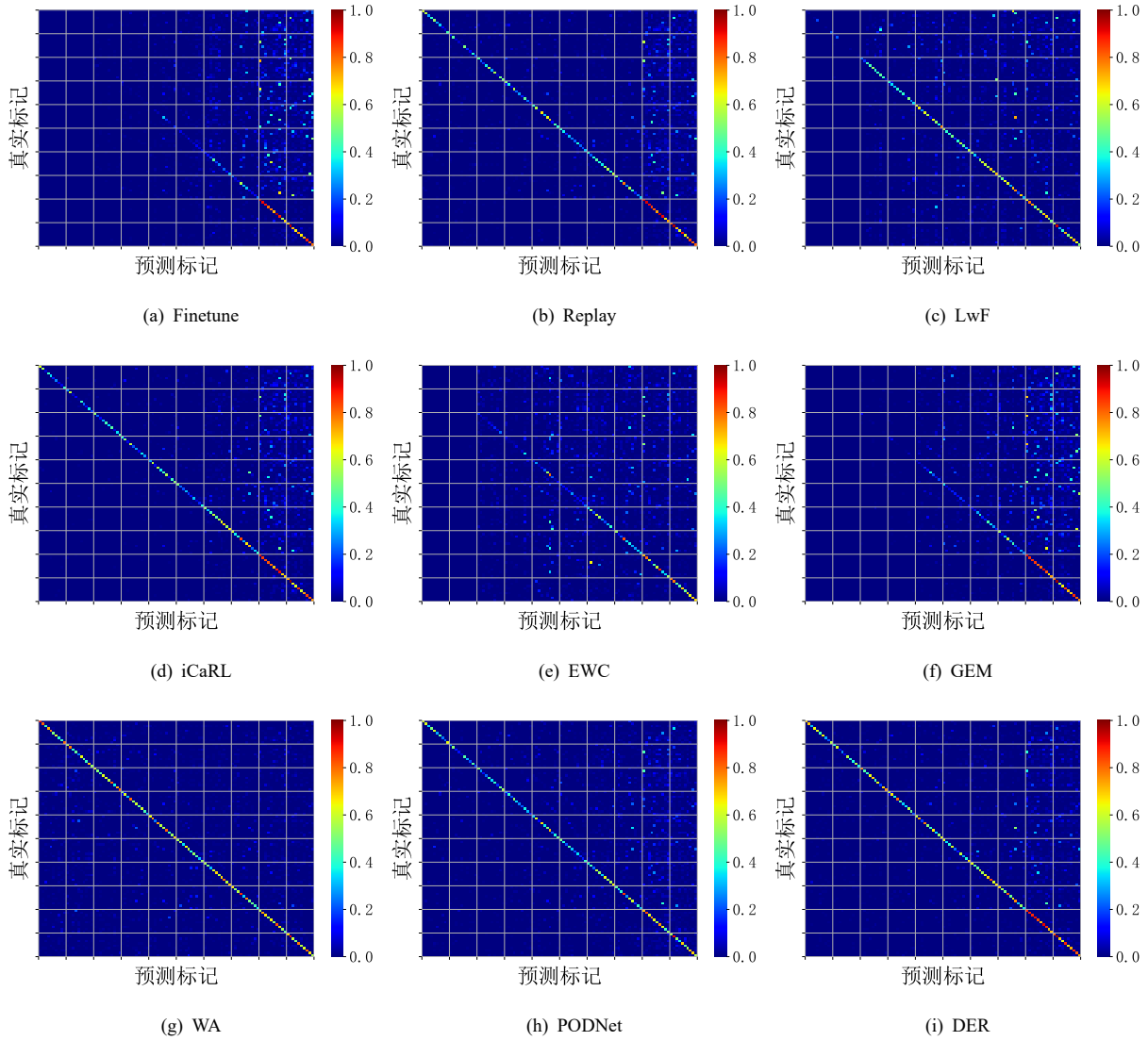
图8 不同类别增量学习算法在 CIFAR100 数据集上预测结果的混淆矩阵
