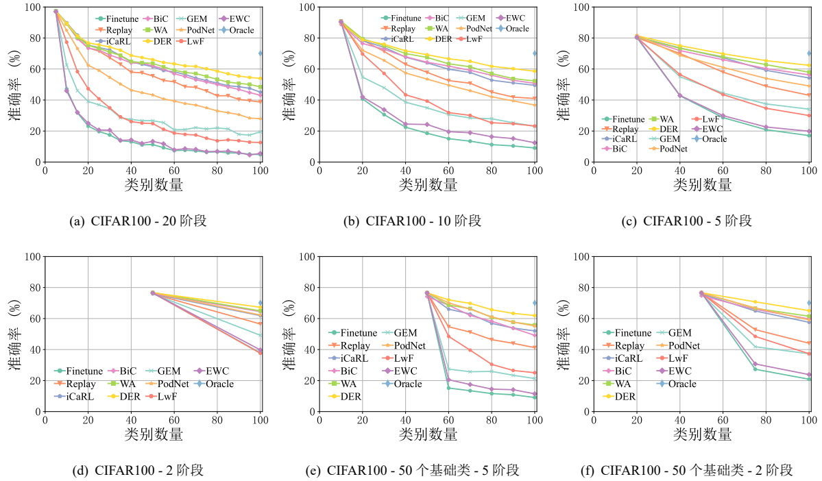
图 4 增量学习算法在 CIFAR100 数据集上的性能对比
