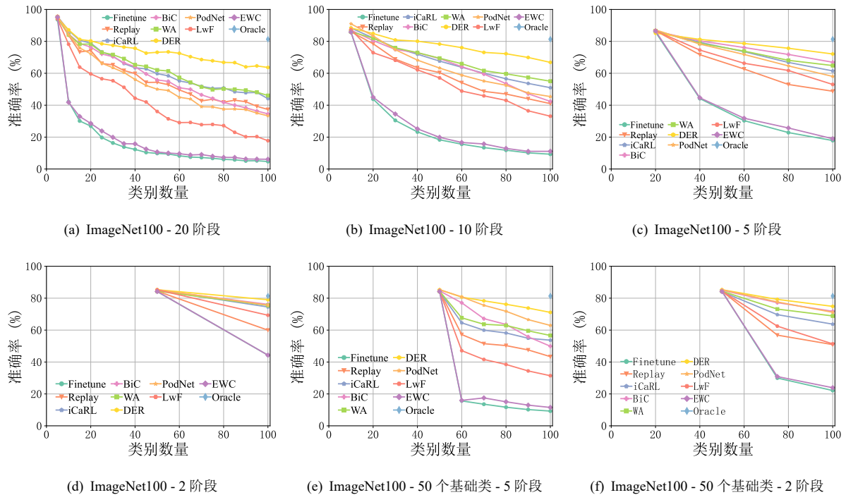
图 5 增量学习算法在 ImageNet100 数据集上的 Top-1 准确率
